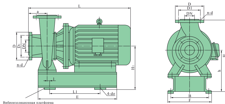
Виброизоляционная платформа
